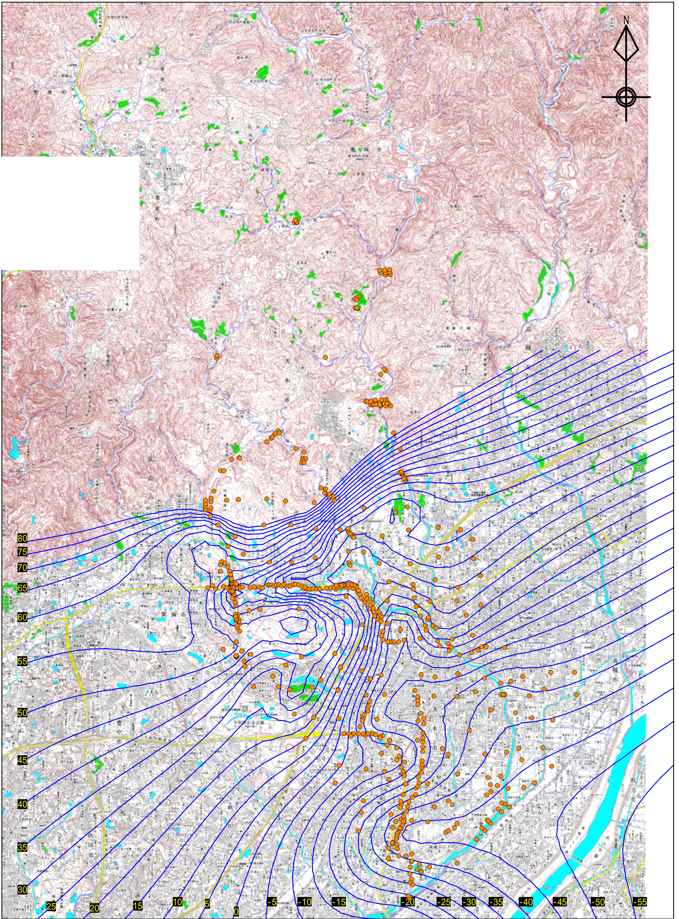
図 洪積層下面コンター図 ( S = 1 : 50,000 )
