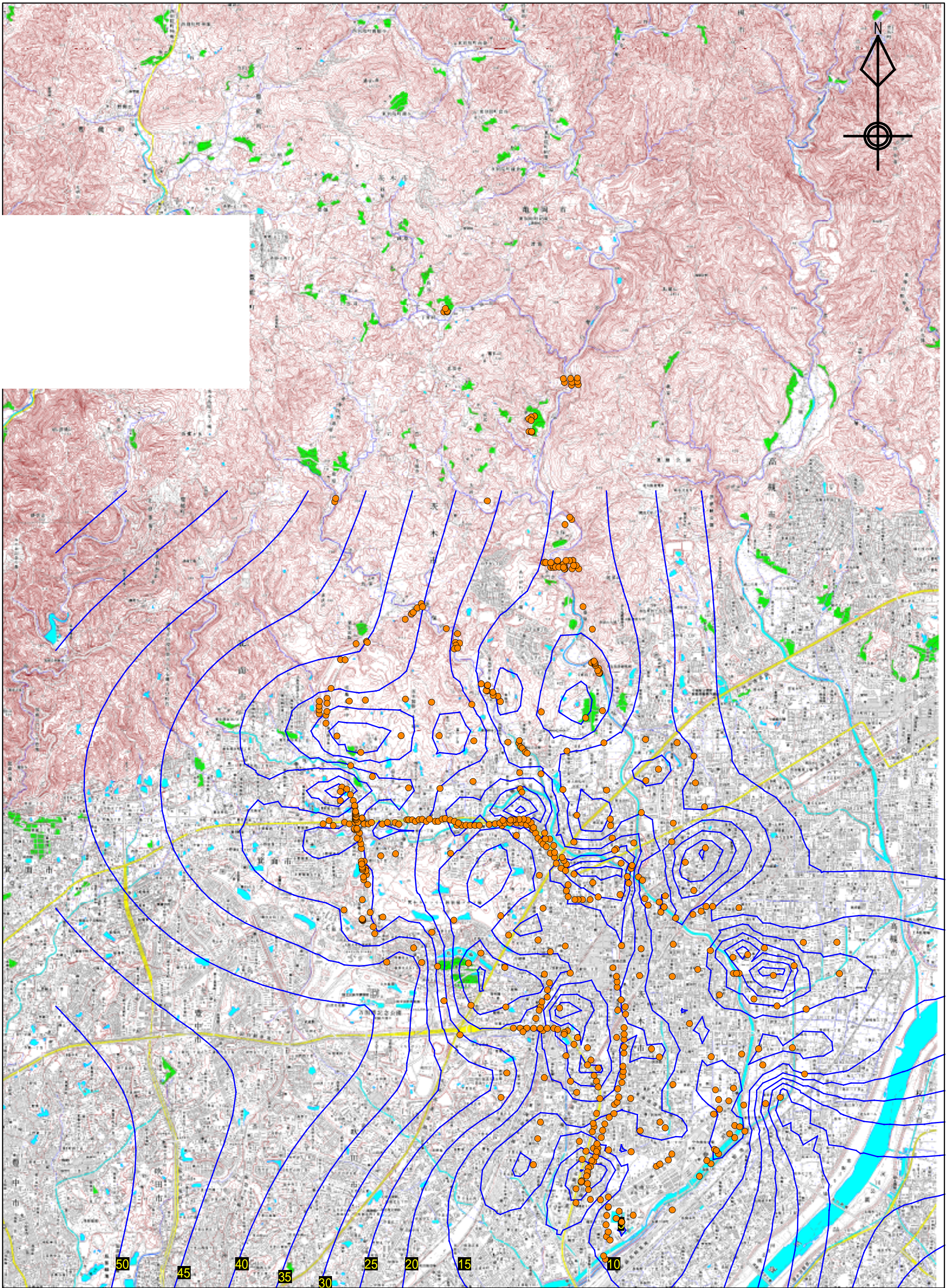
図 洪積層層厚コンター図 ( S = 1 : 50,000 )
