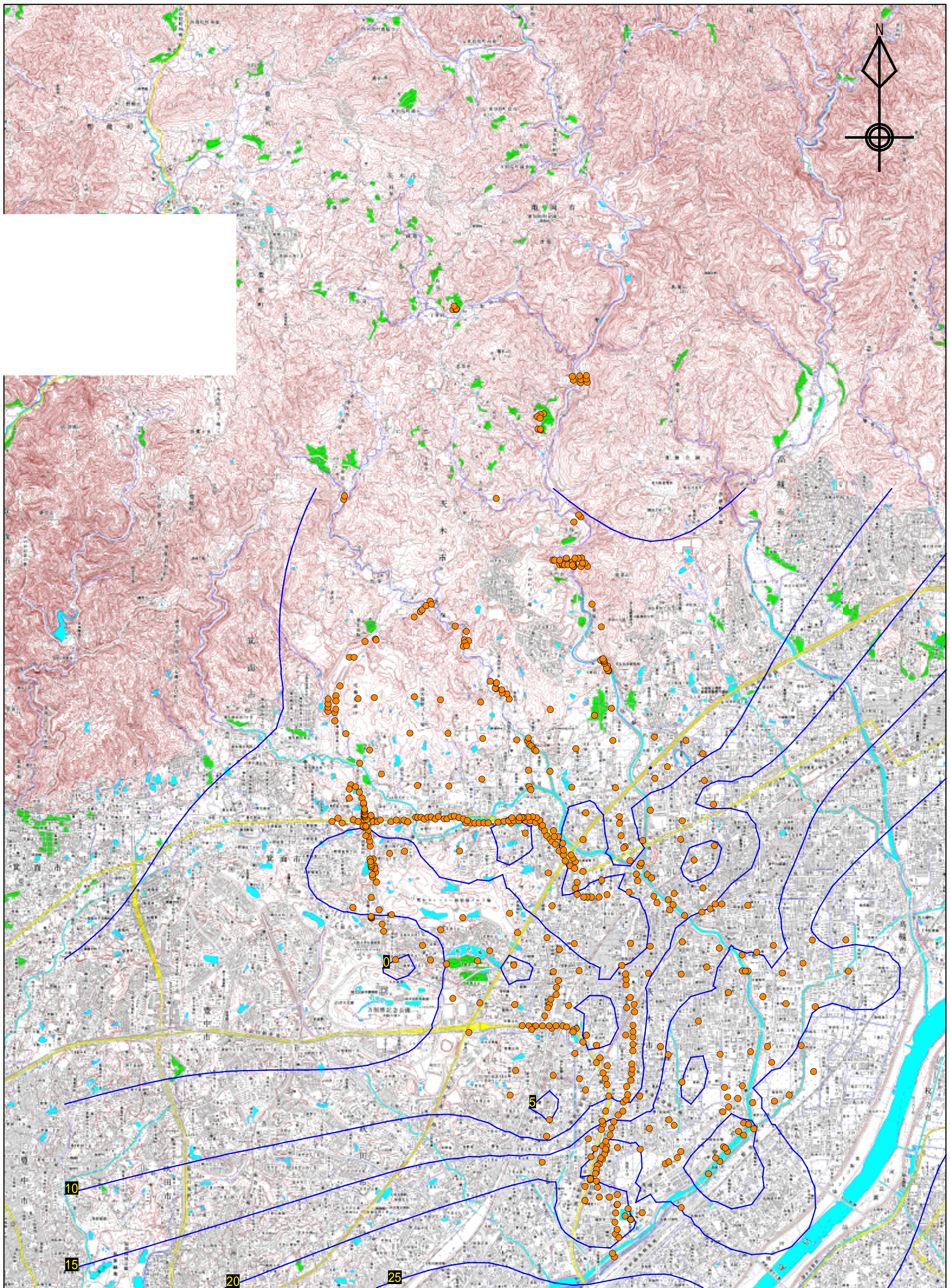
図 沖積層層厚コンター図 ( S = 1 : 50,000 )
